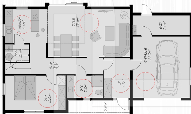
Plan 1. etasje
