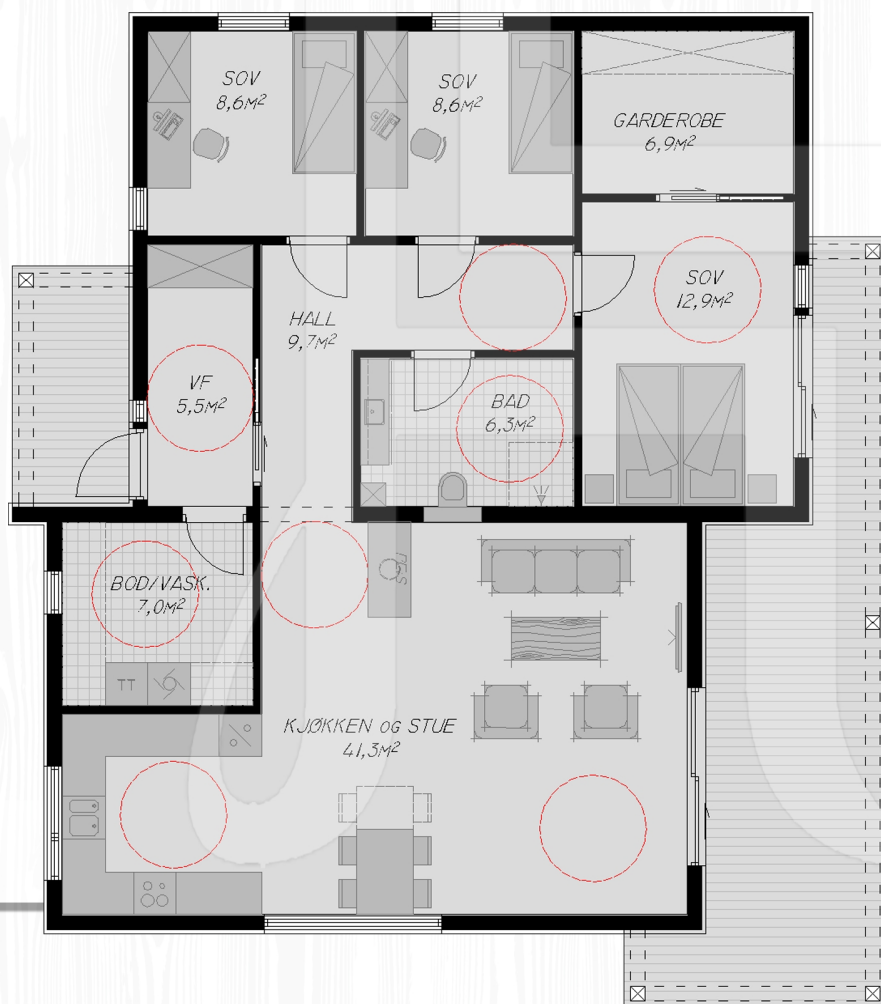
Plan 1. etasje
